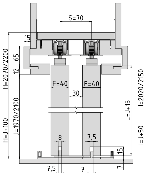
Horizontální řez pouzdra NORMA PARALLEL s dřevěným dveřním křídlem tloušťky 40 mm
